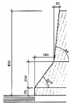
Fig. 7: «New Jersey» profile
